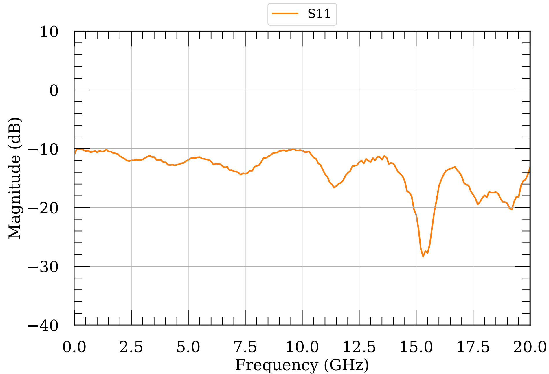
LNA S-params module089
